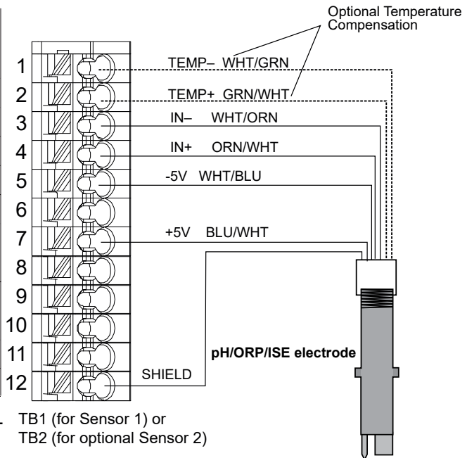
Figura 9 Cablaggio dell'input del sensore pH/ORP/ISE
