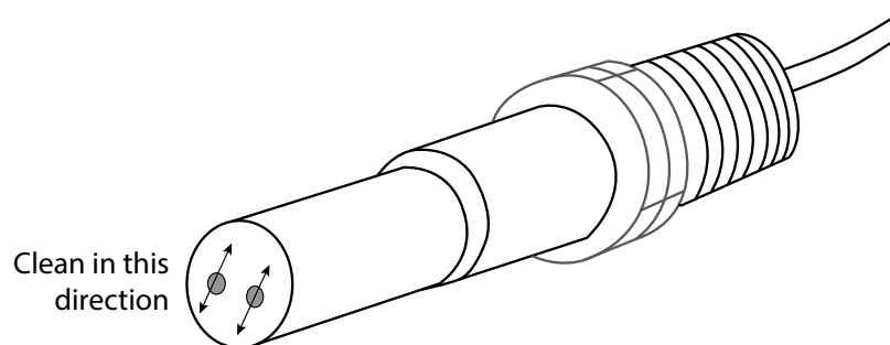
Figura 20 Pulizia dell'elettrodo
