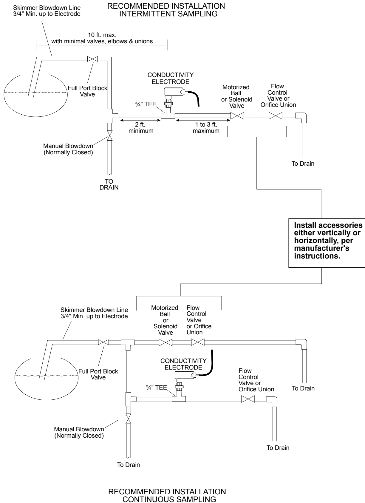
Abbildung 4: Typische Installation – Kessel
