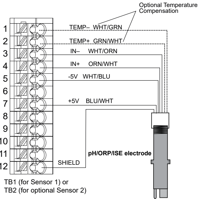
Abbildung 9: Eingangsverdrahtung des pH-/ORP-/ISE-Sensors
