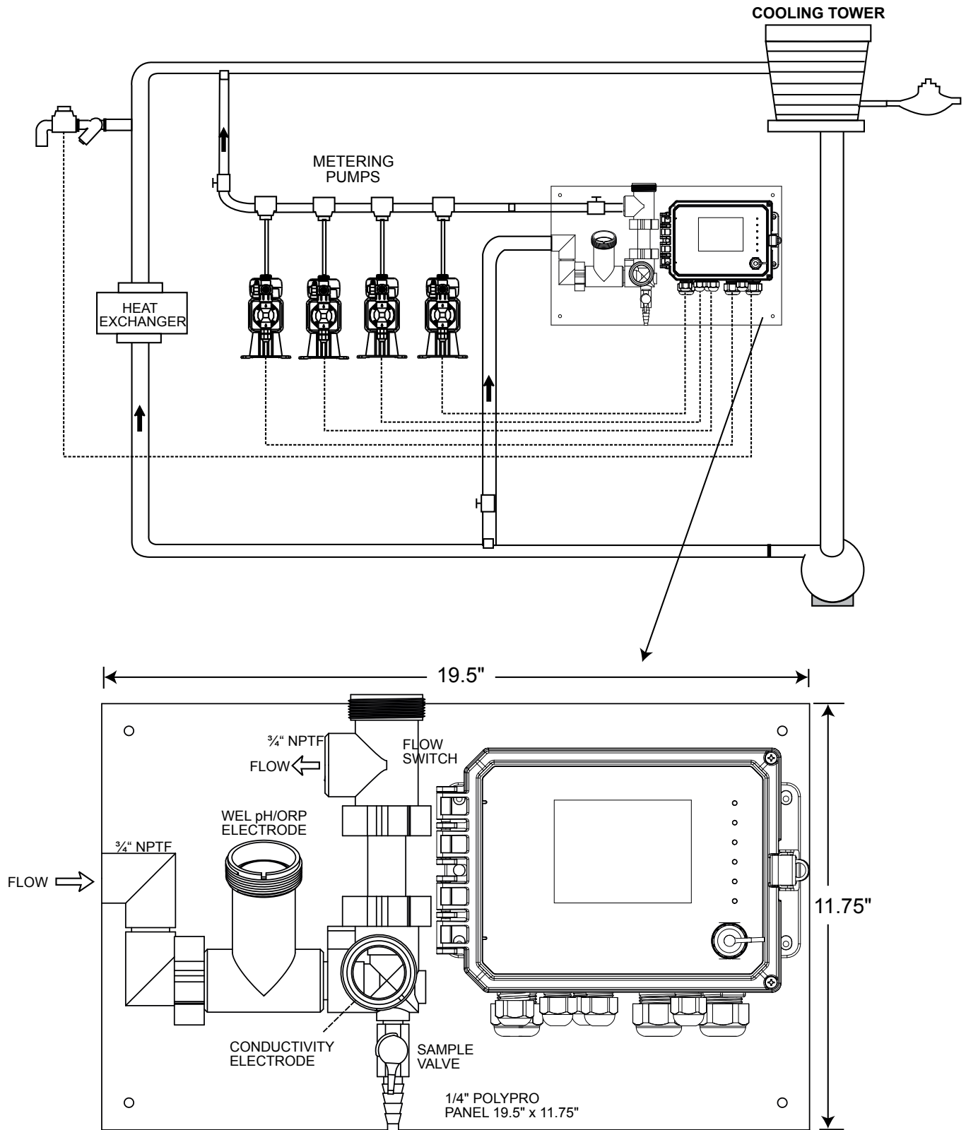
Abbildung 1: Typische Installation – Kühlturm
