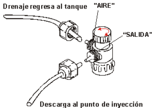
Figura 6 Tubería de Venteo de Aire
