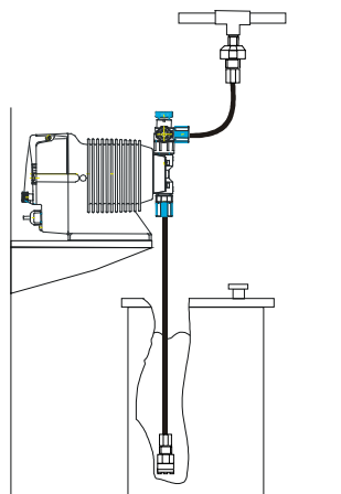
7 Figura 2 Montaje en Estante
