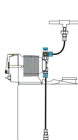
Figura 3 Montaje en Tanque
