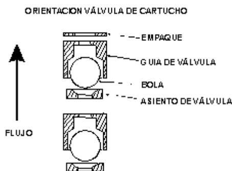
Orientación de la Válvula de Cartucho
