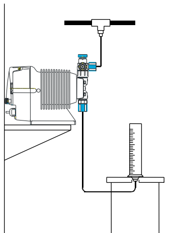
Figura 8 Calibración
