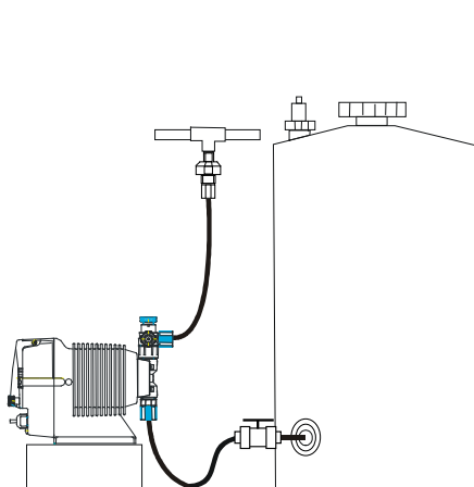
Figura 1 Succión Positiva Recomendada para líquidos que pueden generar burbujas.
