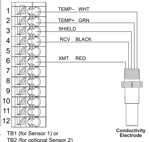
图 7 接触电导率传感器输入接线
