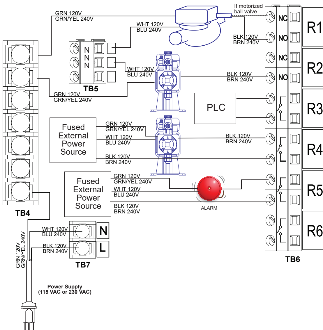
图 15 W610 交流电源和继电器输出接线
