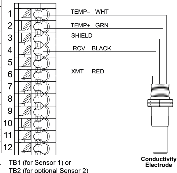
Figura 7 Fiação de entrada do sensor de condutividade por contato
