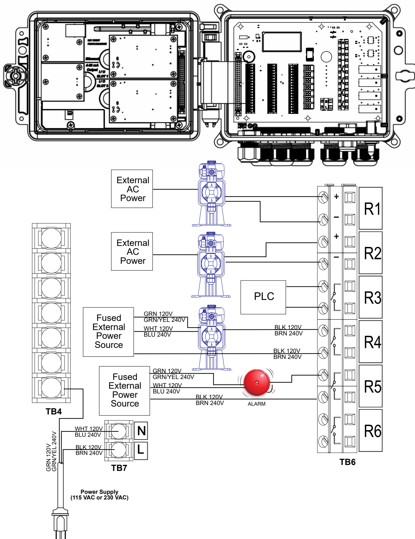
Figura 16 Fiação da saída do relé e alimentação CA W620
